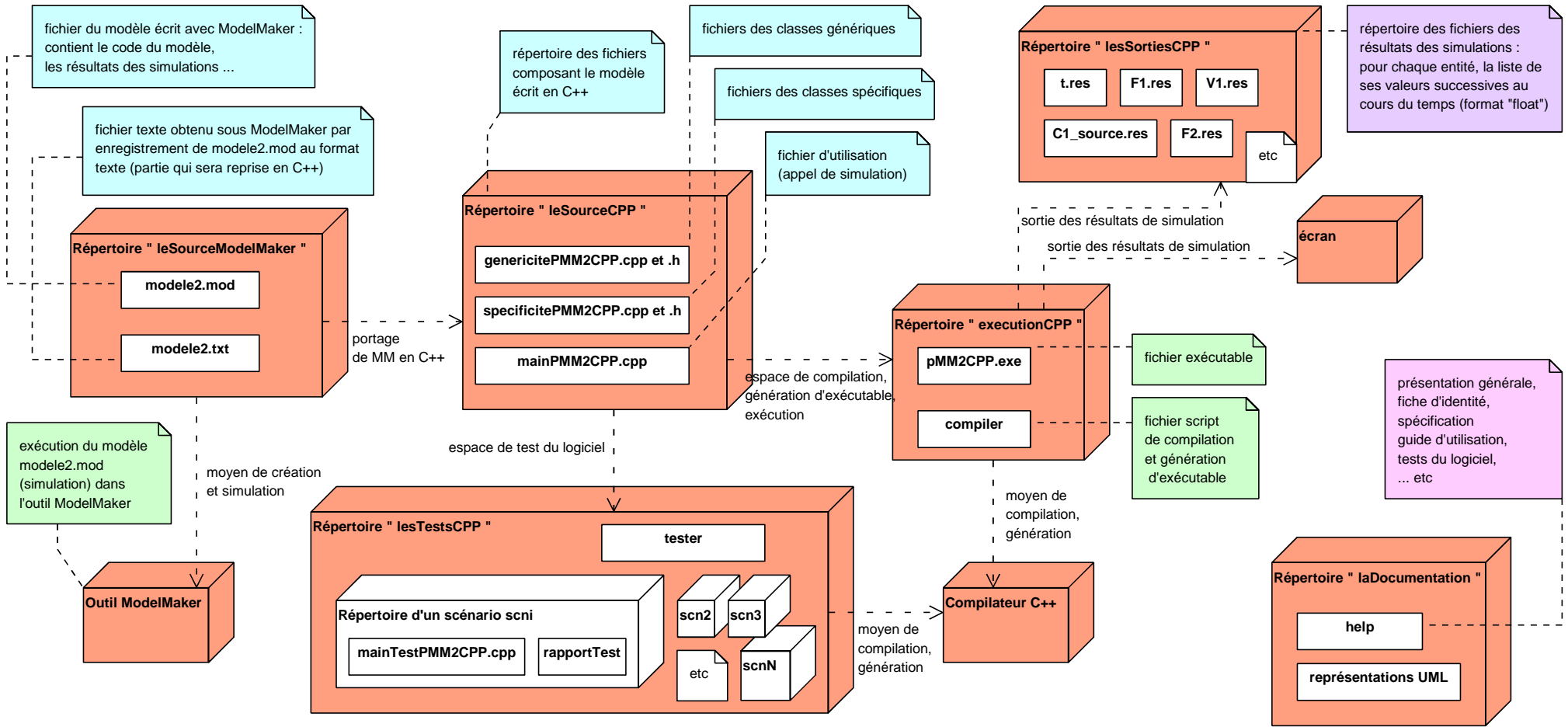
Diagramme de déploiement portageMM2CPP
