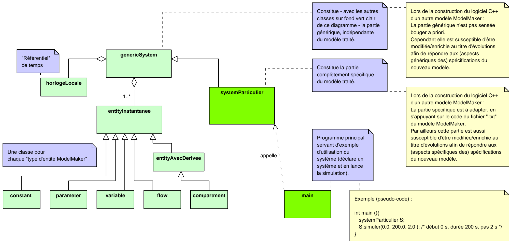
Diagramme des classes du code C++
